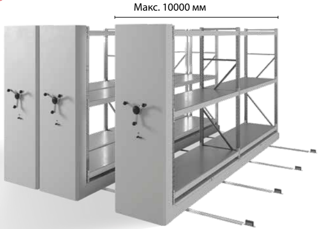
МТА со стеллажами MS PRO
